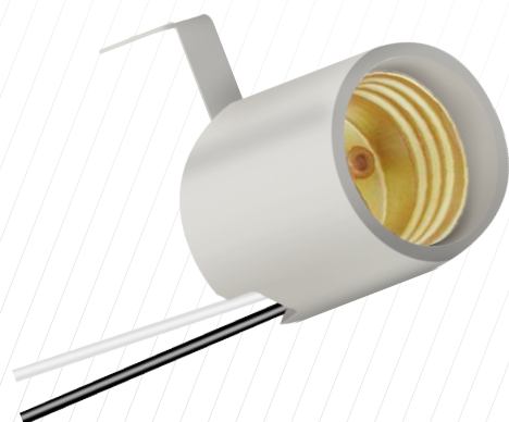
● SOCKET PORCELANA CON ESCUADRA E26 clave S00692
