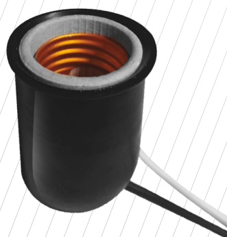
● SOCKET PORCELANA/ CUBIERTA DE PLÁSTICO clave S00699
